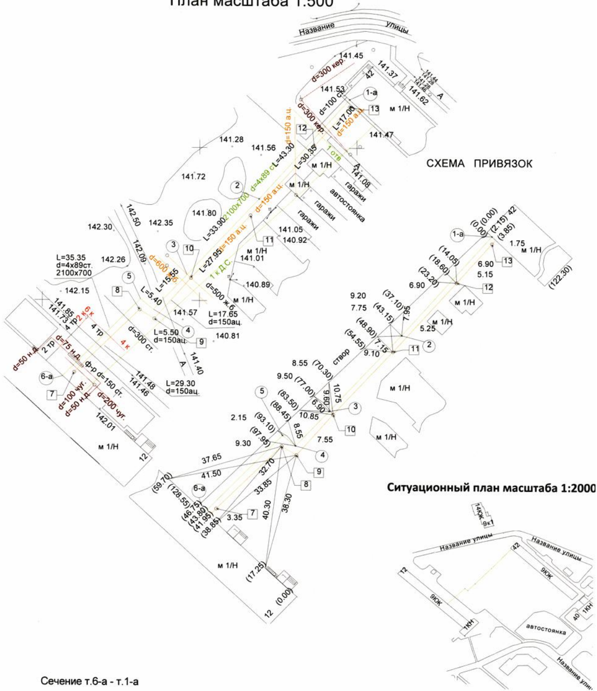
План масштаба 1:500
