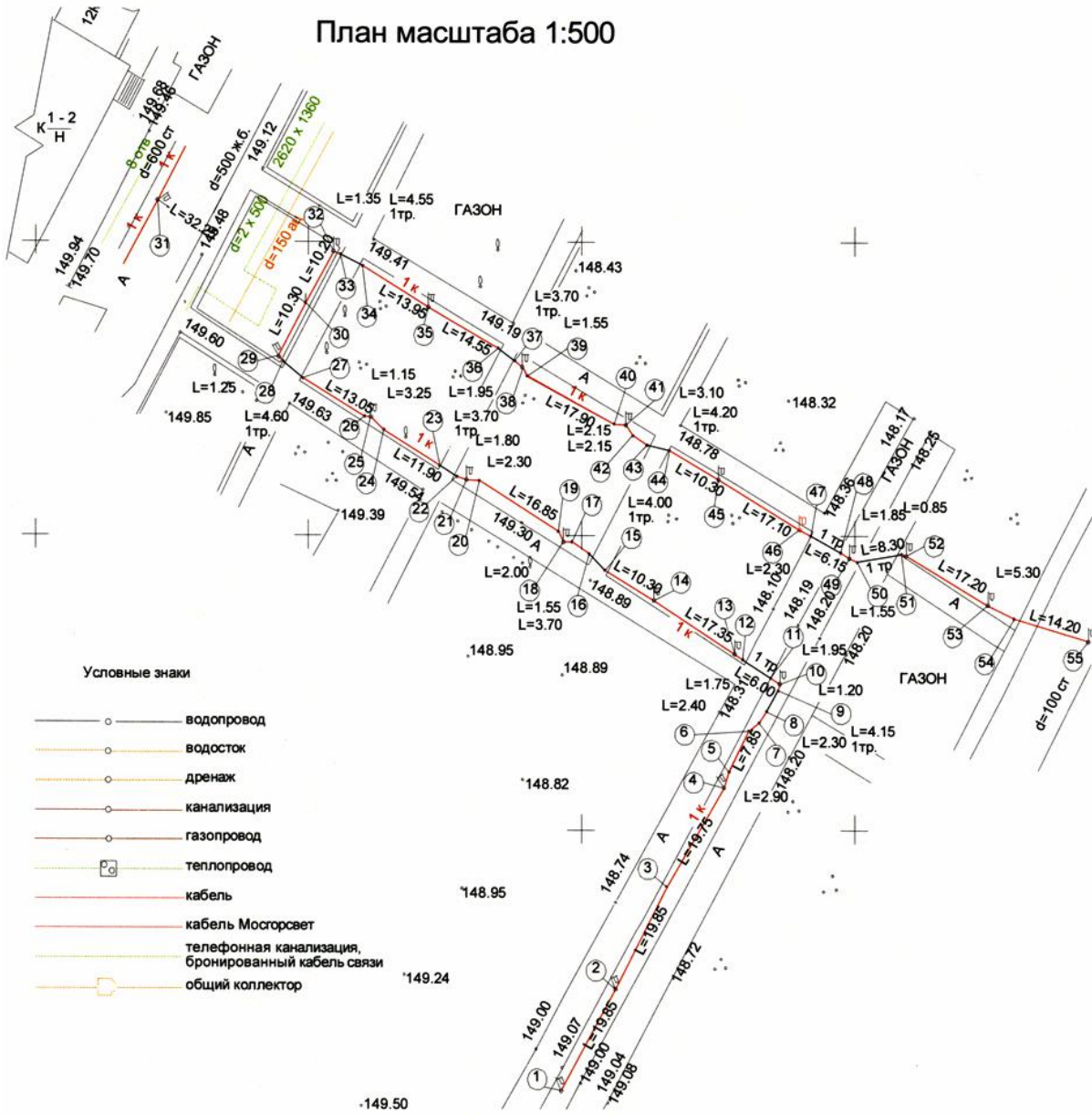
Рисунок Ж.7, лист 1
