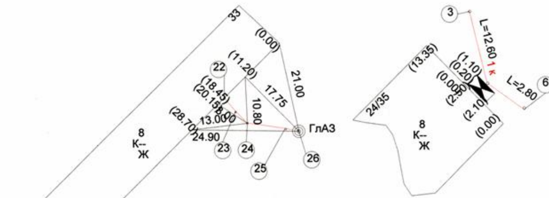
СХЕМА ПРИВЯЗОК т.3-т.11
