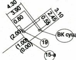
Камера в т.ВК сущ.
