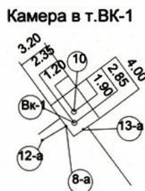
Камера в т.ВК сущ.
