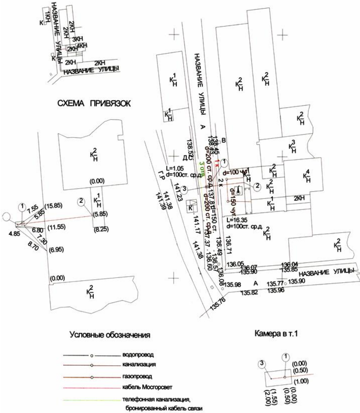
Рисунок Ж.4, лист 1
