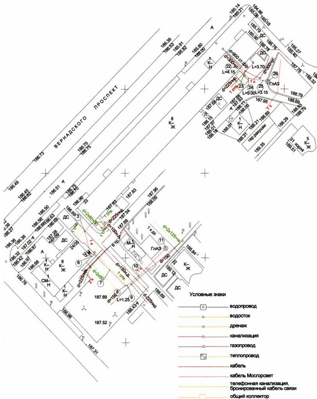
План масштаба 1:500
