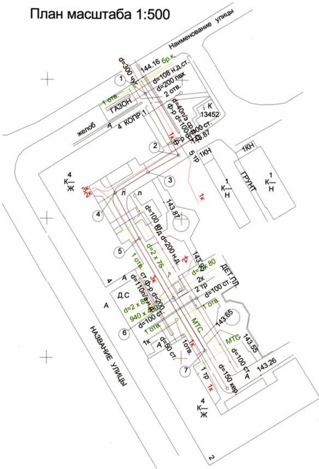
Рисунок Ж.9, лист 1
