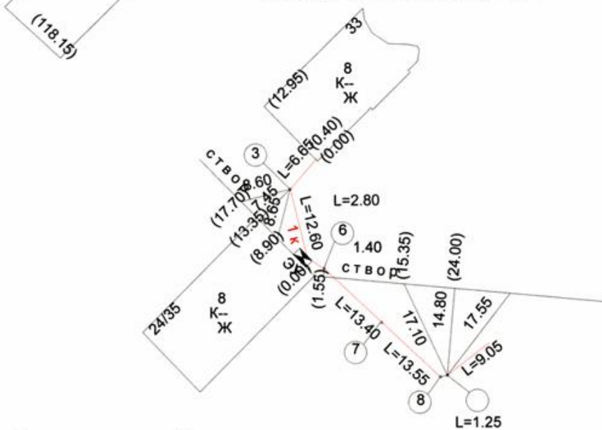
Ситуационный план масштаба 1:2000
