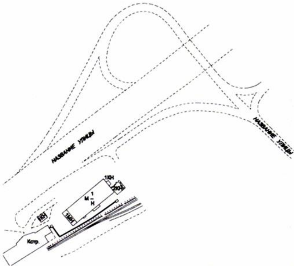
Ситуационный план масштаба 1:2000
